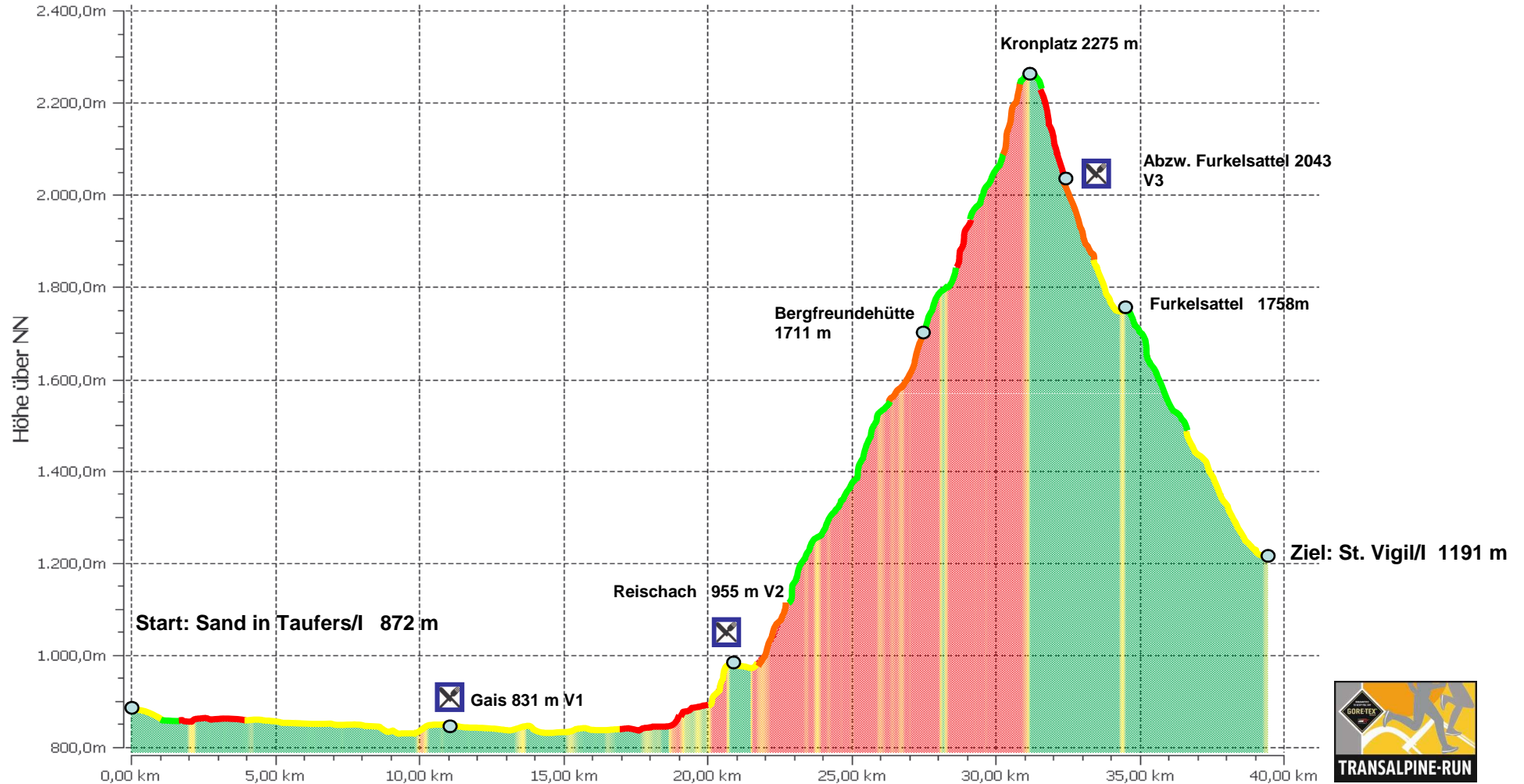
Höhenprofil
